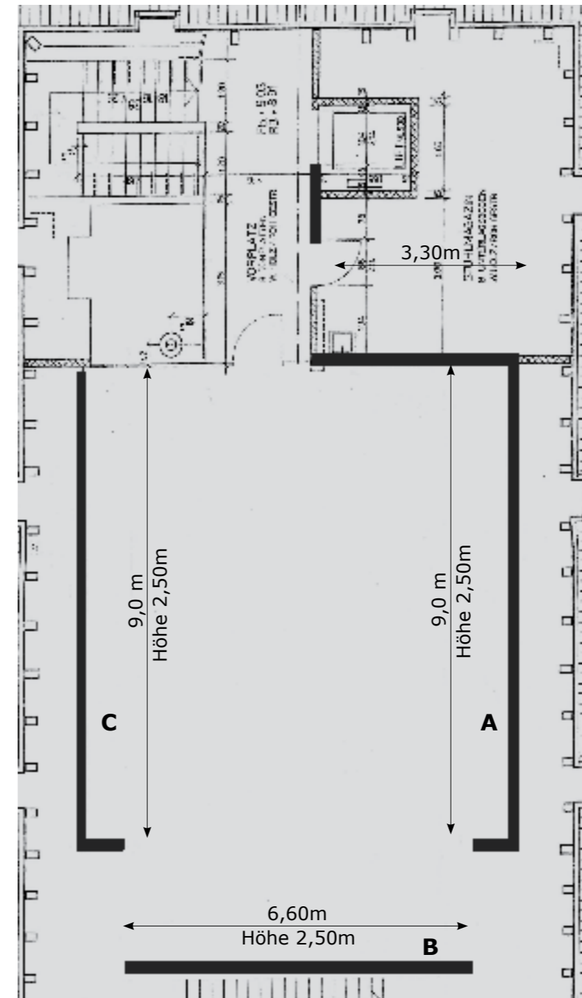
OBERE ETAGE GRUNDRISS
