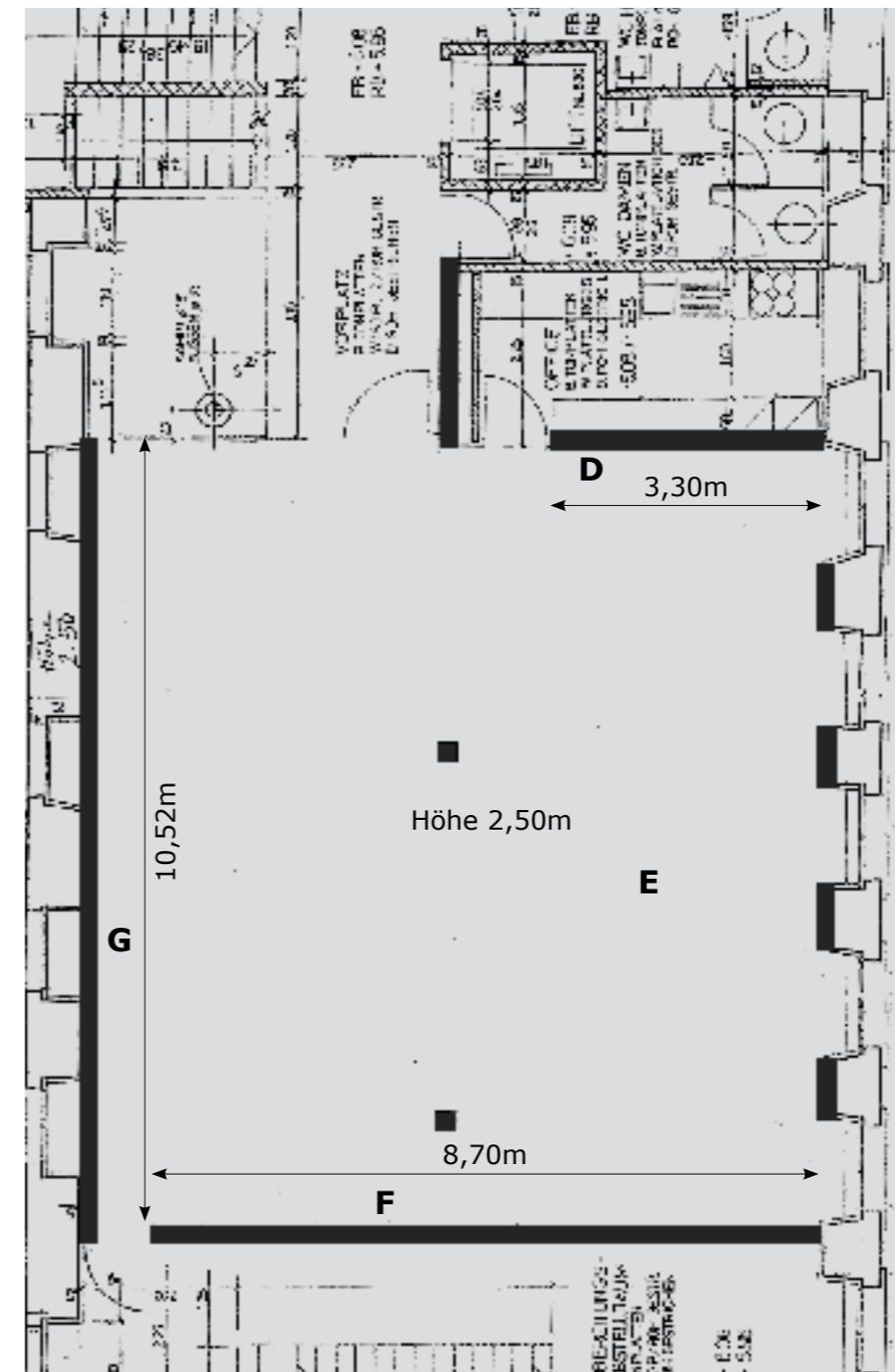
UNTERE ETAGE GRUNDRISS
